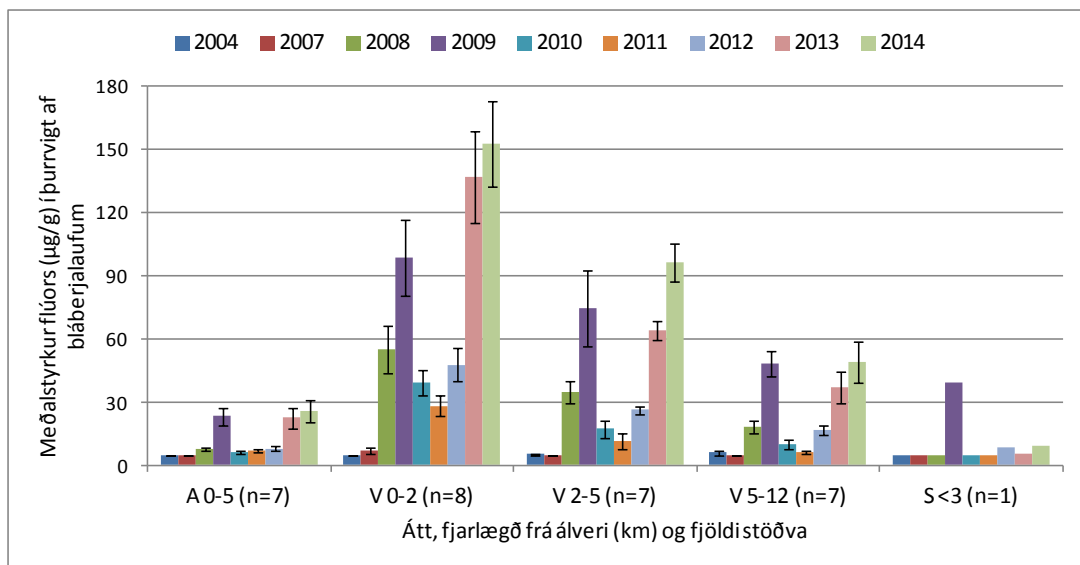
Mynd 38. Dreifingarmynstur flúors í bláberjalyngi frá árinu 2004 (bakgrunnsgildi) til ársins 2014. Áttir A-austur, V-vestur og S-suður og fjarlægð frá reykháfi álvers. Fjöldi sýna er gefinn upp í sviga. Einnig er sýnd staðalskekkja meðaltalanna.
